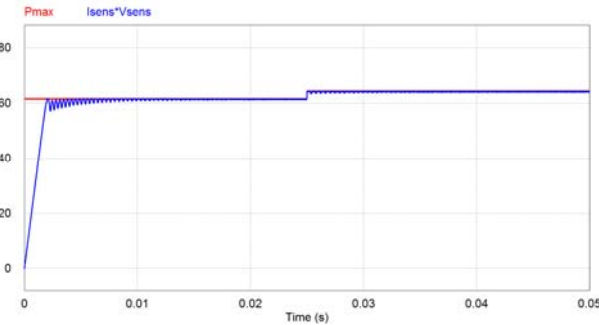
(d) Proposed INC in temperature 25 °C → 15 °C
