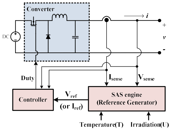
Fig. 1. Solar array simulator.
